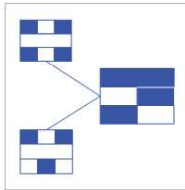
Diagrama PERT
