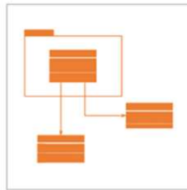
Clase UML
