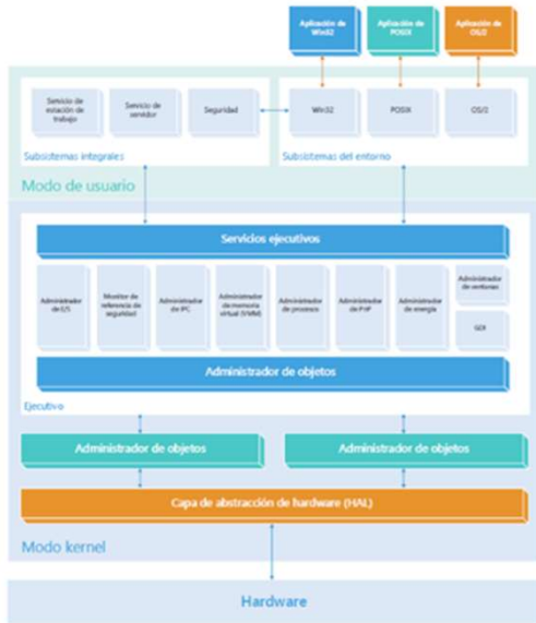
Arquitectura de Windows NT
